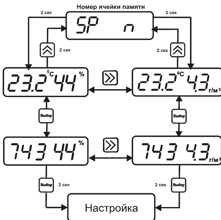
Рисунок 5.4 Режим РАБОТА ИВТМ-7М5, ИВТМ-7М5-3
