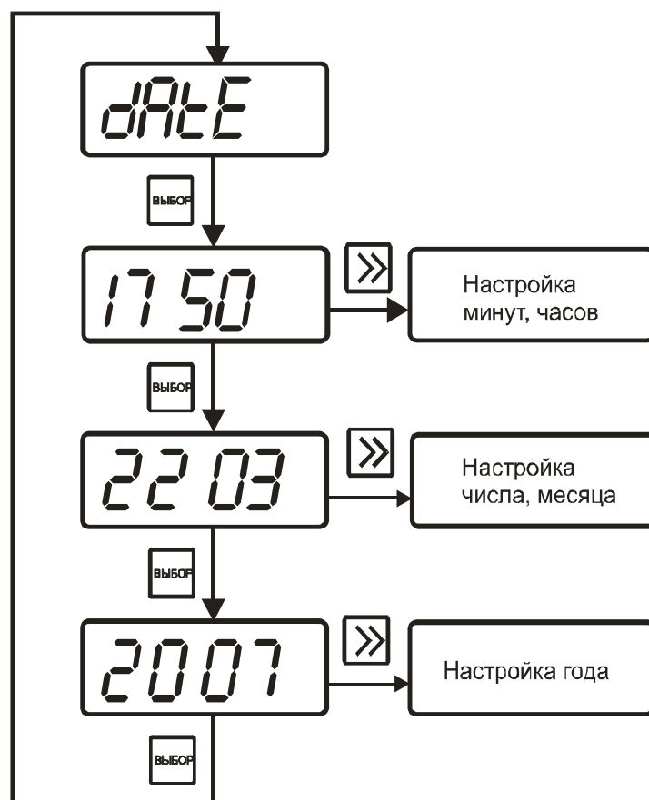
Рисунок 5.22 Установка часов реального времени
