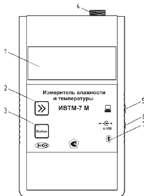
Рисунок 3.5 Внешний вид измерительного блока ИВТМ-7М7-1, ИВТМ-7М7-2
