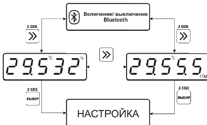
Рисунок 5.8 Режим РАБОТА ИВТМ-7М7-1
