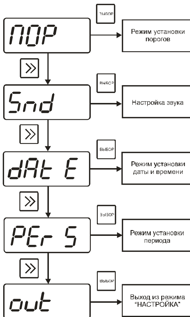
Рисунок 5.17 Схема режима НАСТРОЙКА ИВТМ-7М6-1, ИВТМ-7М6-2
