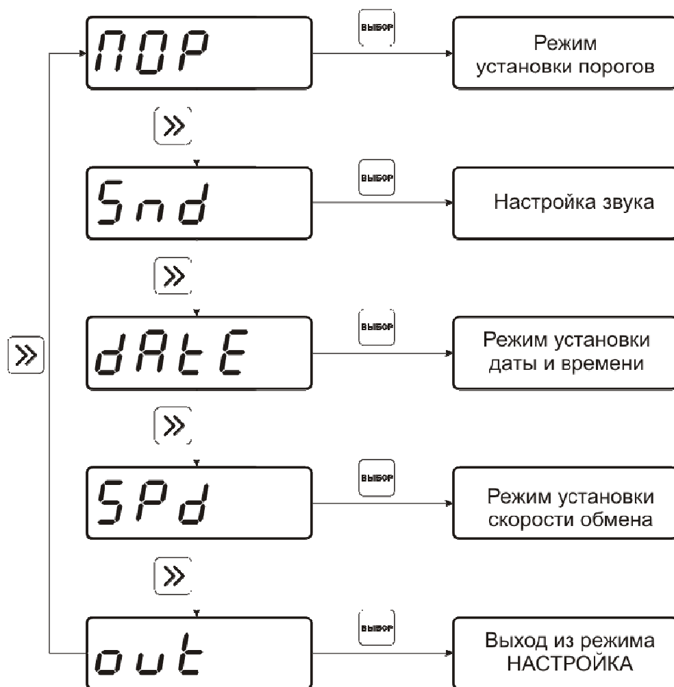
Рисунок 5.20 Схема режима НАСТРОЙКА ИВТМ-7М7-1, ИВТМ-7М7-2
