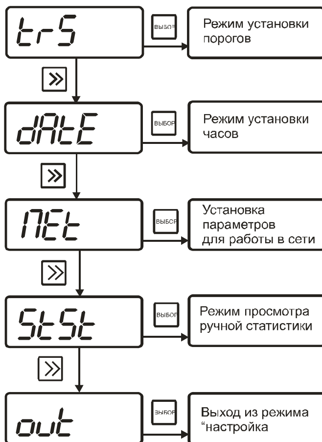
Рисунок 5.10 Схема режима НАСТРОЙКА ИВТМ-7М1, ИВТМ-7М2, ИВТМ-7М3, ИВТМ-7М5, ИВТМ-7М5-3
