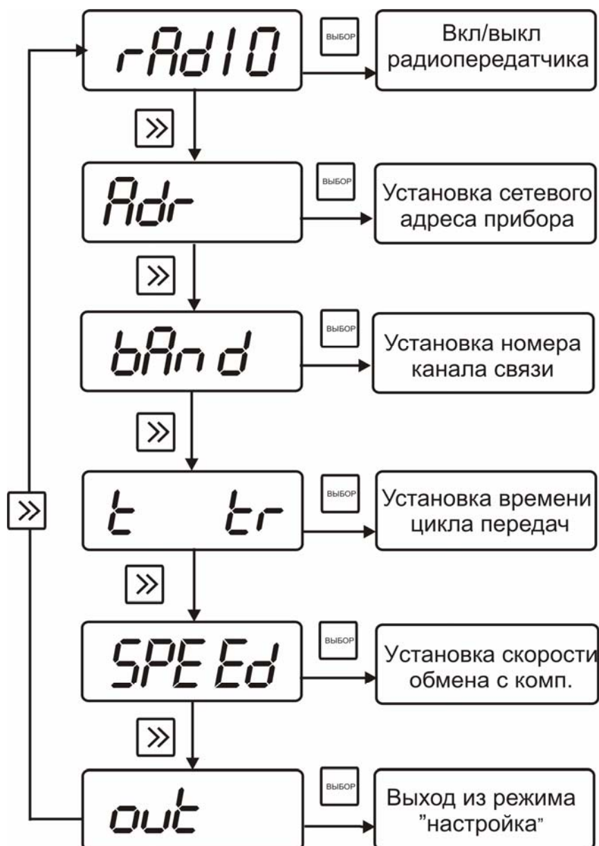
Рисунок 5.16 Схема режима НАСТРОЙКА ИВТМ-7М4
