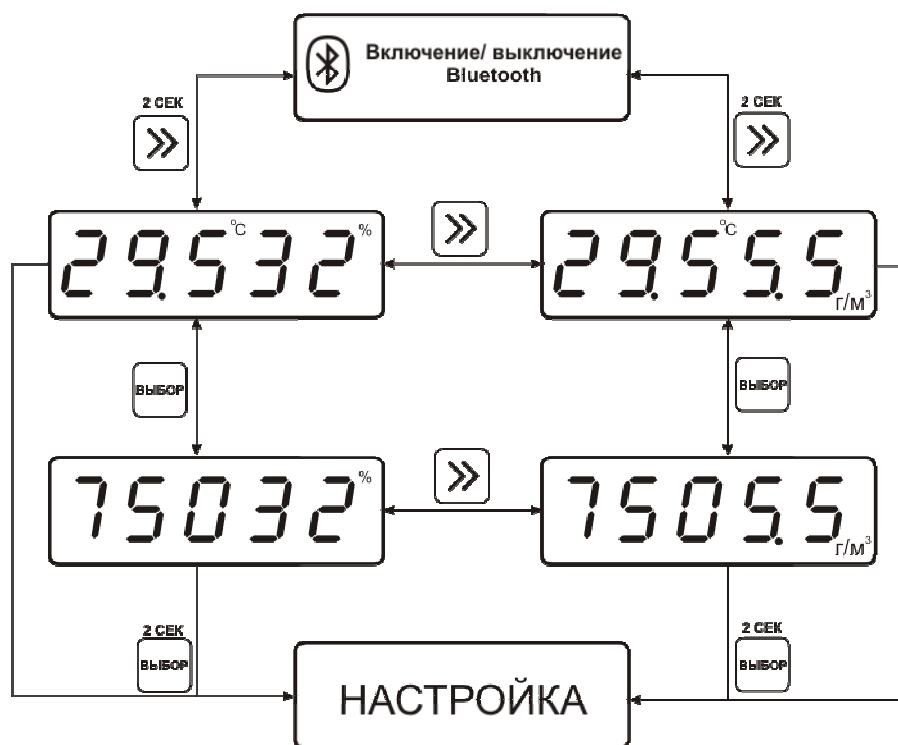
Рисунок 5.9 Режим РАБОТА ИВТМ-7М7-2
