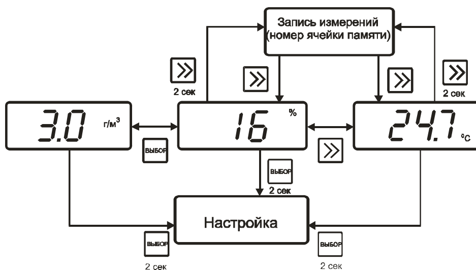
Рисунок 5.1 Режим РАБОТА ИВТМ-7М1
