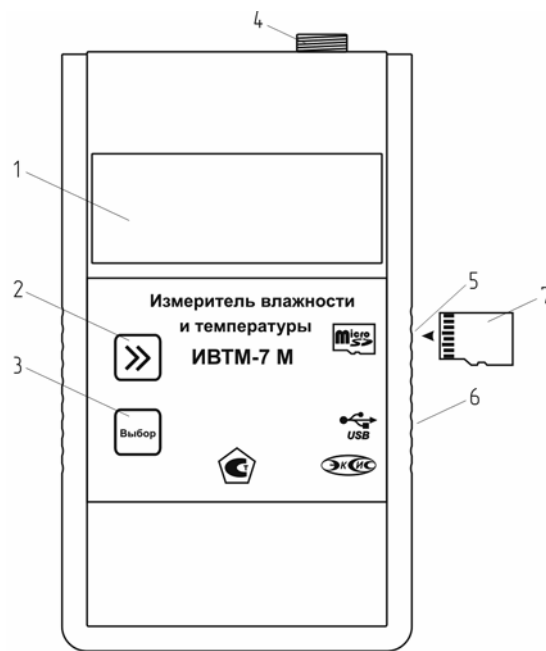
Рисунок 3.4 Внешний вид измерительного блока ИВТМ-7М6-1, ИВТМ-7М6-2
