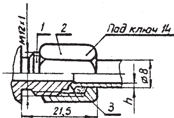
Исполнение 1 для металлических труб
