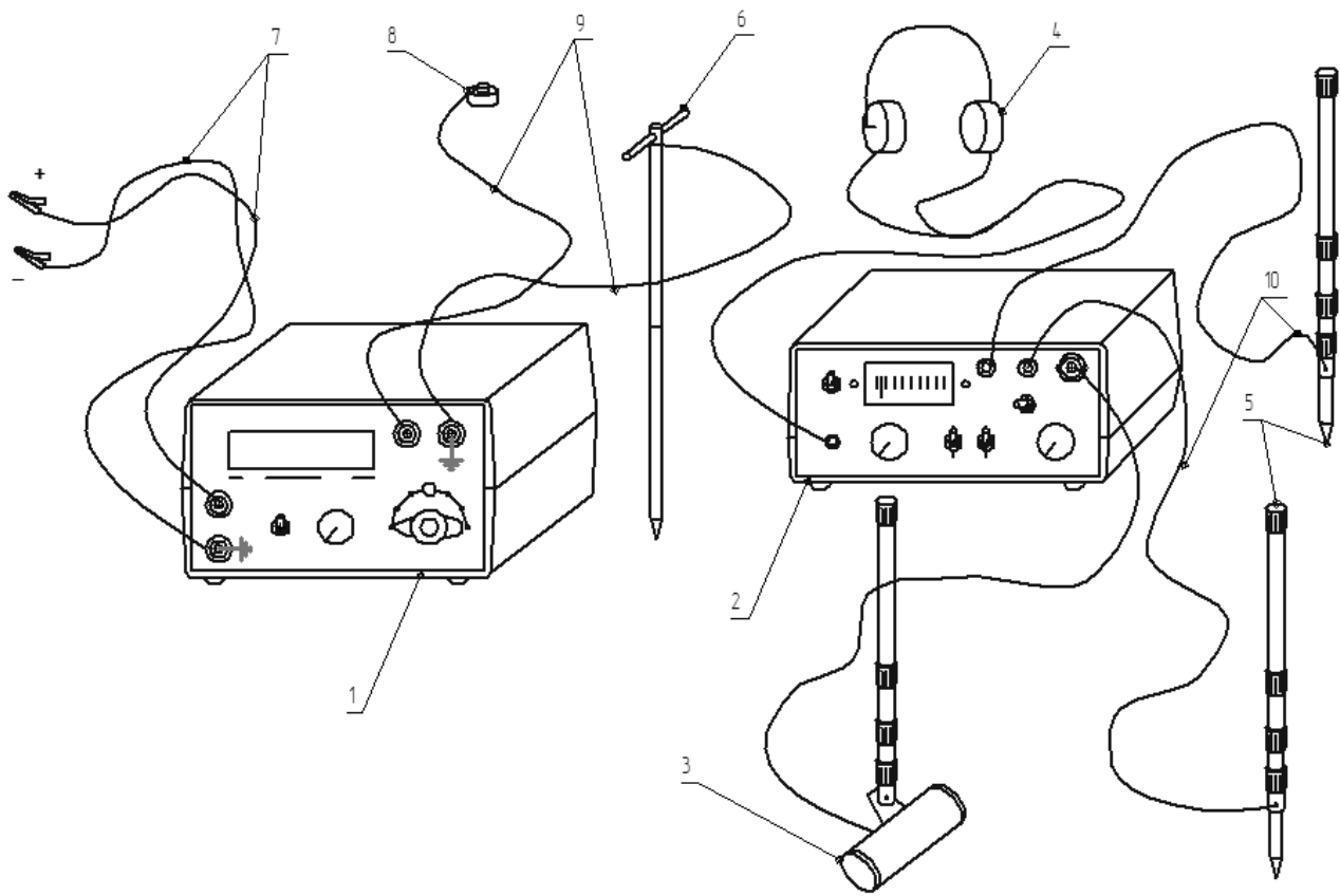
Рис.1. Комплект ИПИ-95К
