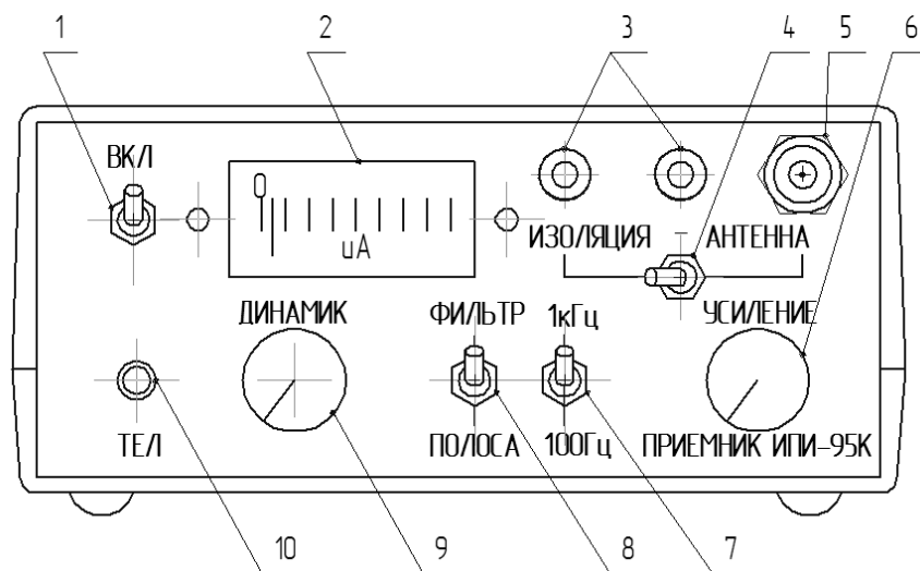
Рис.4. Передняя панель приемника
