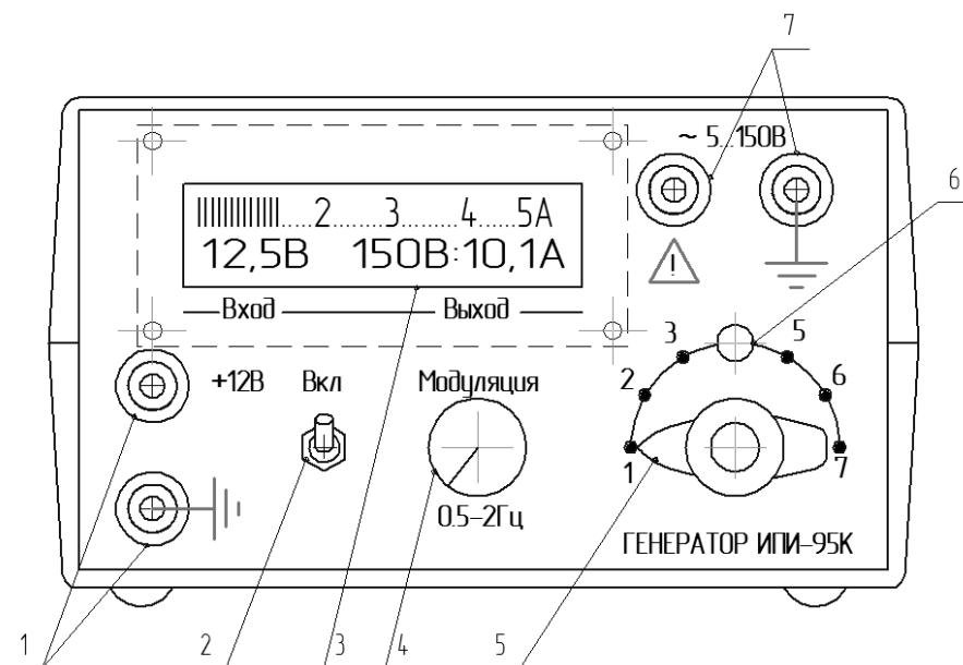
Рис.5. Передняя панель генератора
