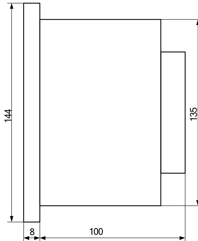
Рис. 1.1 Габаритные размеры щитового варианта указателя положения РПН УП 200-Б
