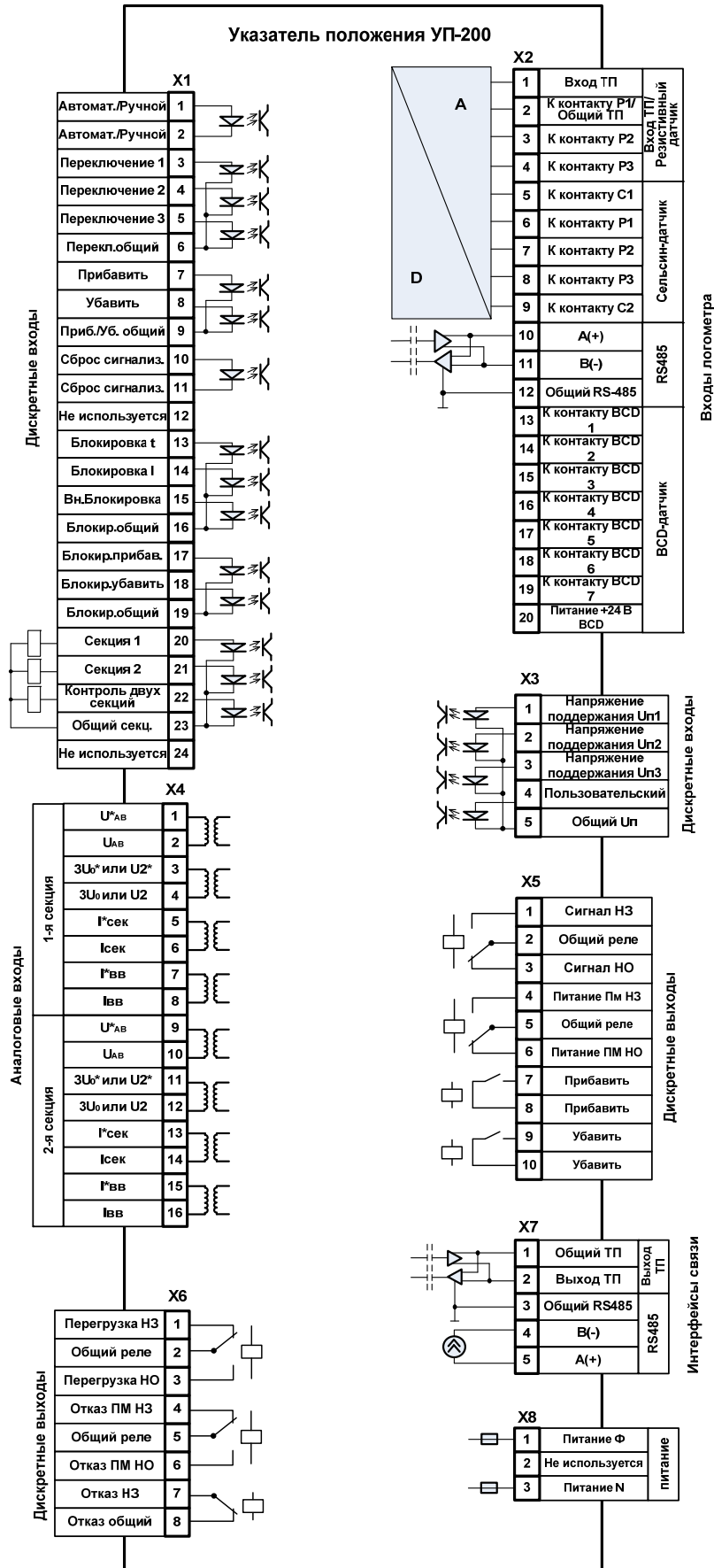
Рис. 3.1 Схема подключения УП 200
