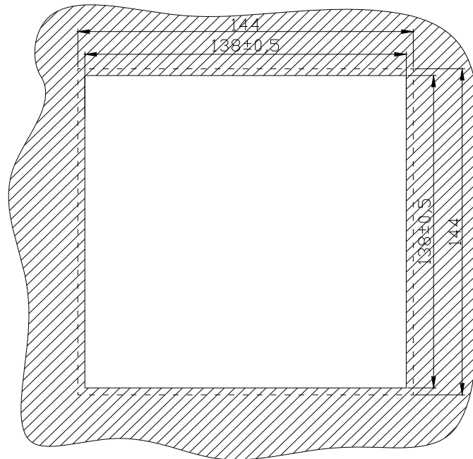
Рис. 2.1 Размеры вырубаемого окна в щите для установки щитового варианта указателя положения УП 200-Б
