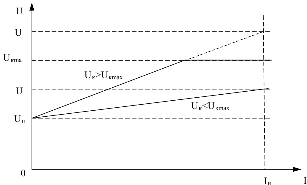
Рис. 1 Зависимость напряжения компенсации от тока нагрузки U_{\text{к}}
