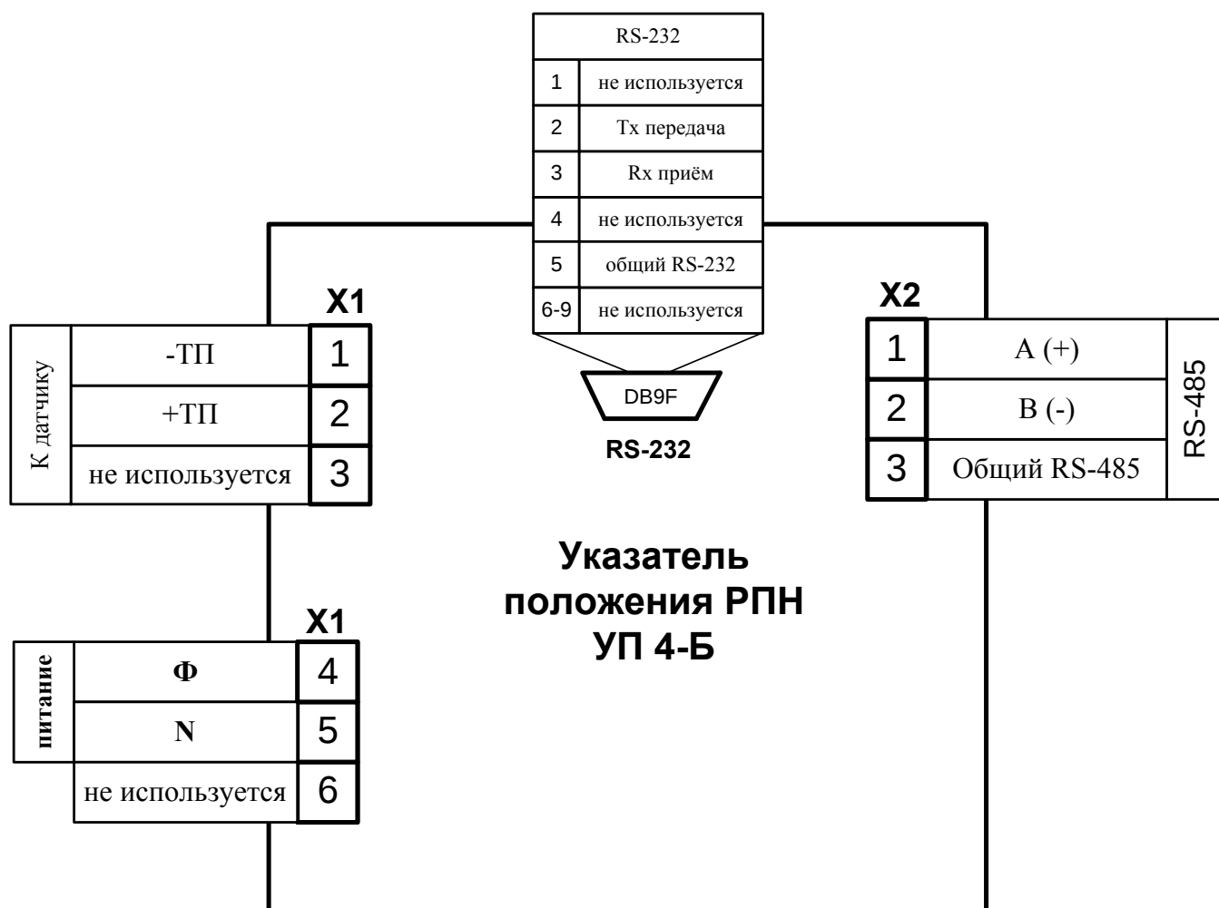
Рис. 3.1 Схема подключения УП 4-Б
