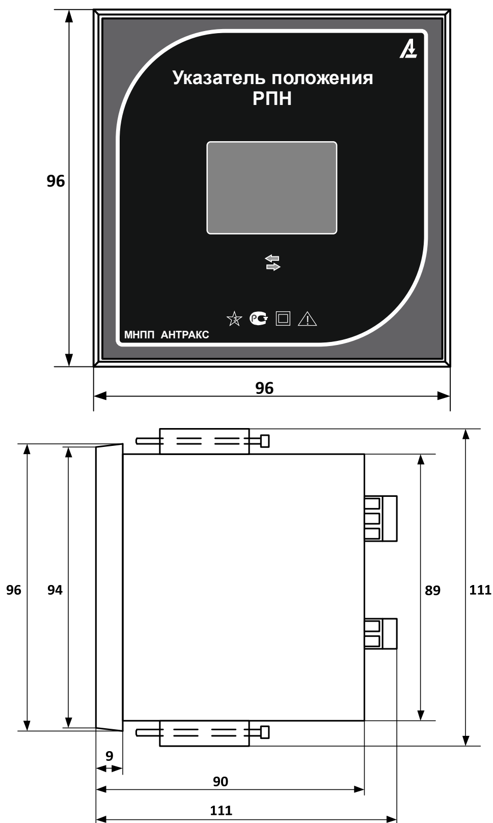
Рис. 1.1 Габаритные размеры щитового варианта указателя положения РПН УП 4-Г
