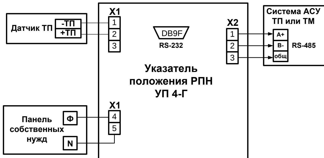
Рис. 4.1 Схема привязки УП 4-Г к приводу типа MZ-2, MZ-4.
