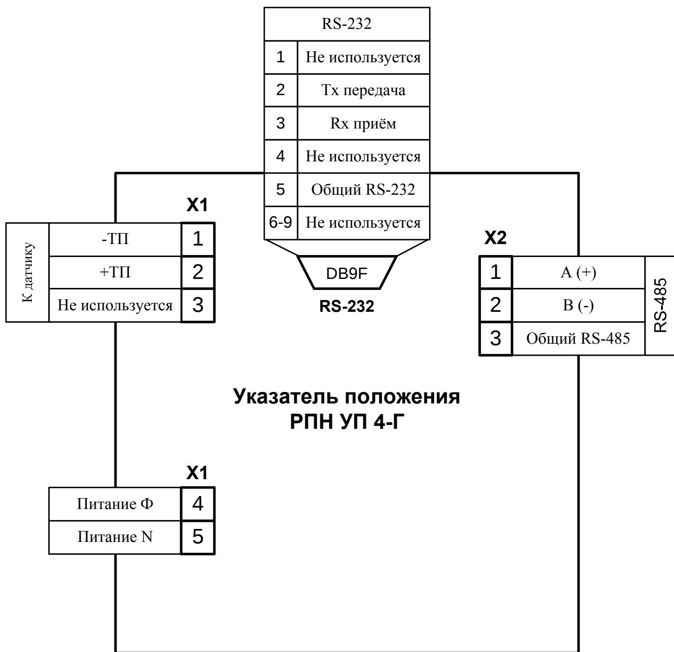
Рис. 3.1 Схема подключения УП 4-Г
