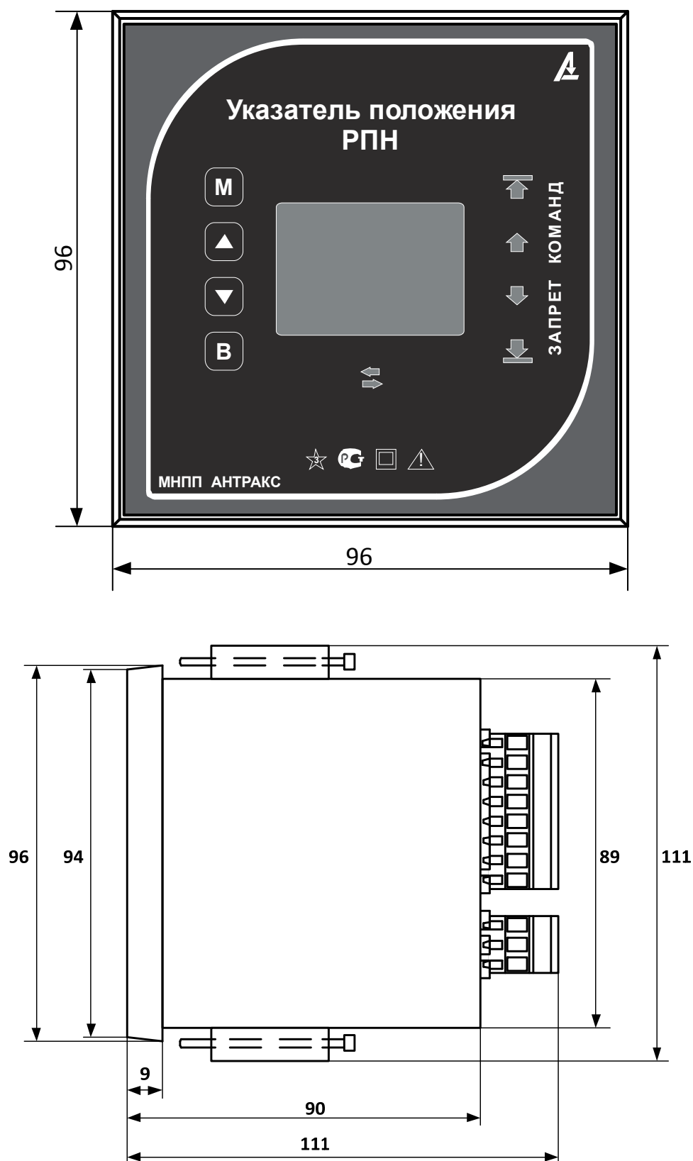
Рис. 1.1 Габаритные размеры щитового варианта указателя положения РПН УП 25-Г
