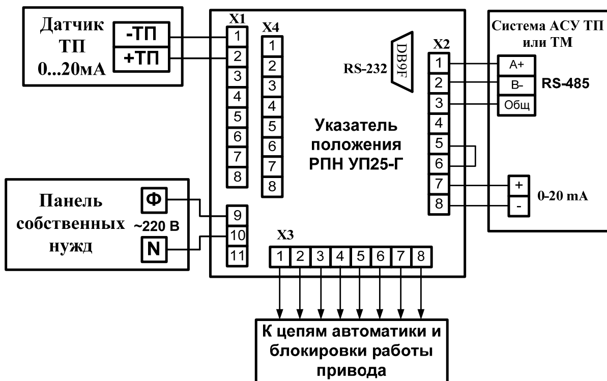
Рис. 4.3 Схема привязки УП 25-Г к датчику «токовая петля» 0-20 мА.
