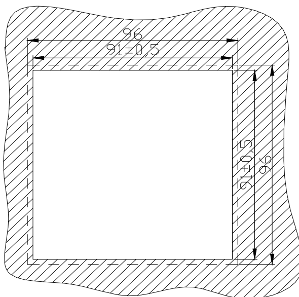
Рис. 2.1 Размеры вырубаемого окна в щите для установки щитового варианта указателя положения УП 25-Г
