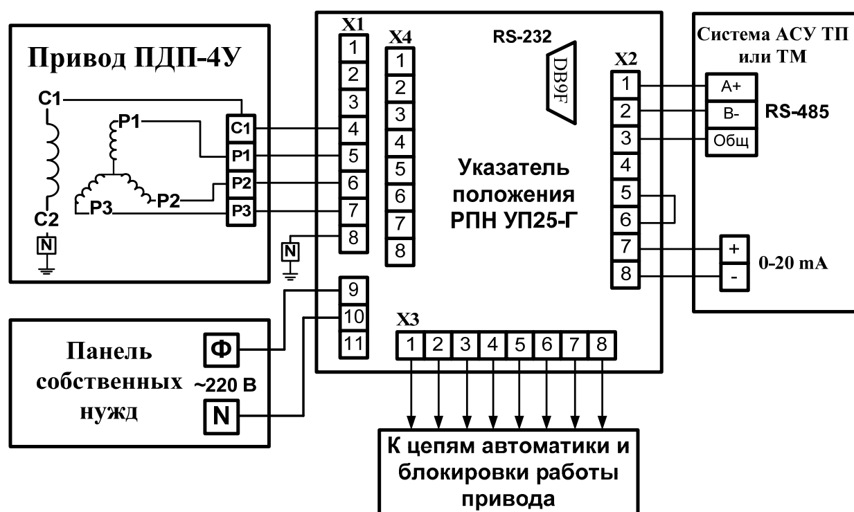
Рис. 4.1 Схемы привязки УП 25-Г к приводу типа ПДП-4У.
