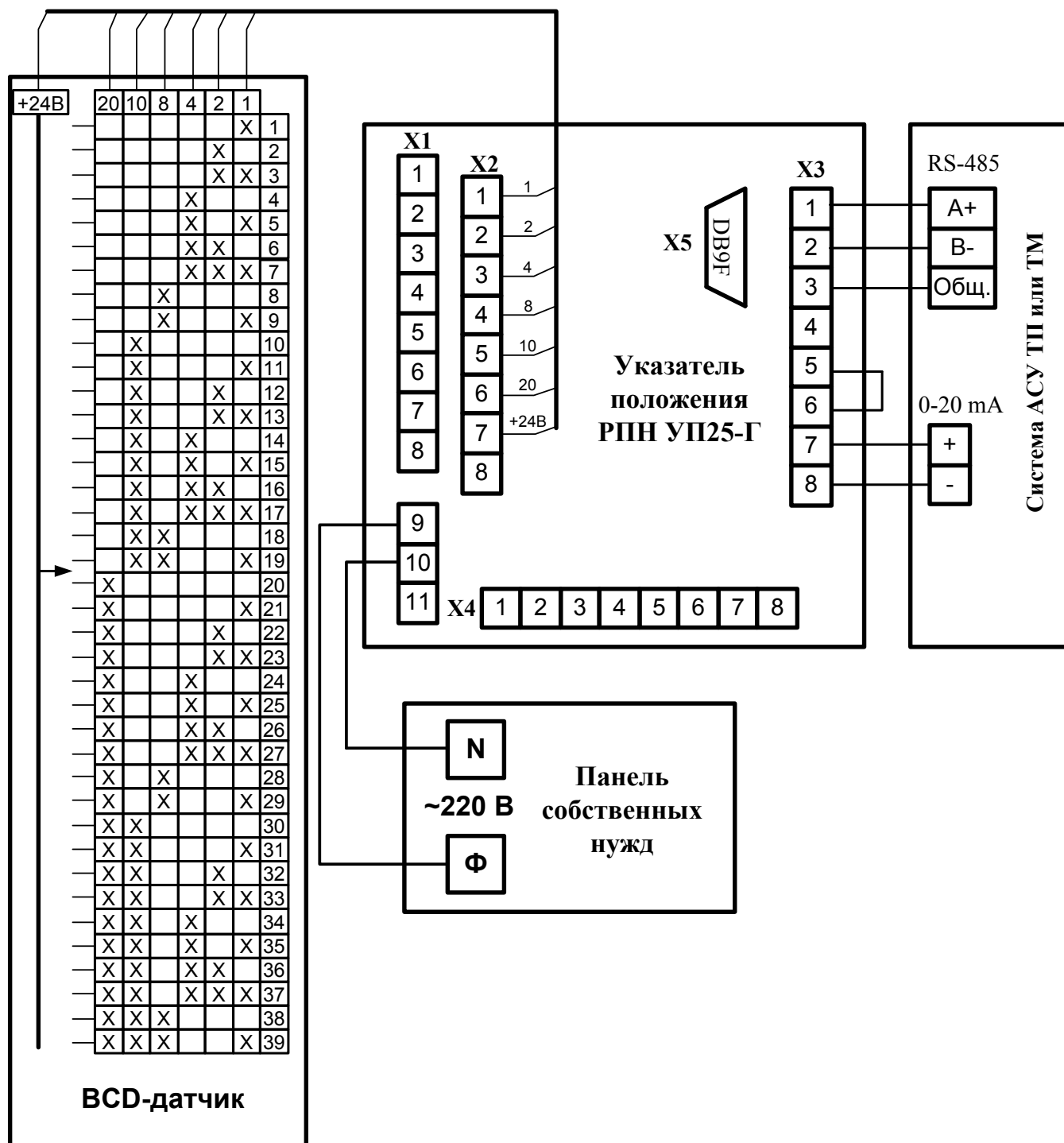
Рис. 4.4 Схема привязки УП 25-Г к BCD-датчику.
