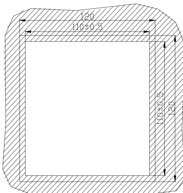
Рис. 2.2 Размеры вырубаемого окна в щите для установки щитового варианта указателя положения УП 25-Г с промежуточной рамкой
