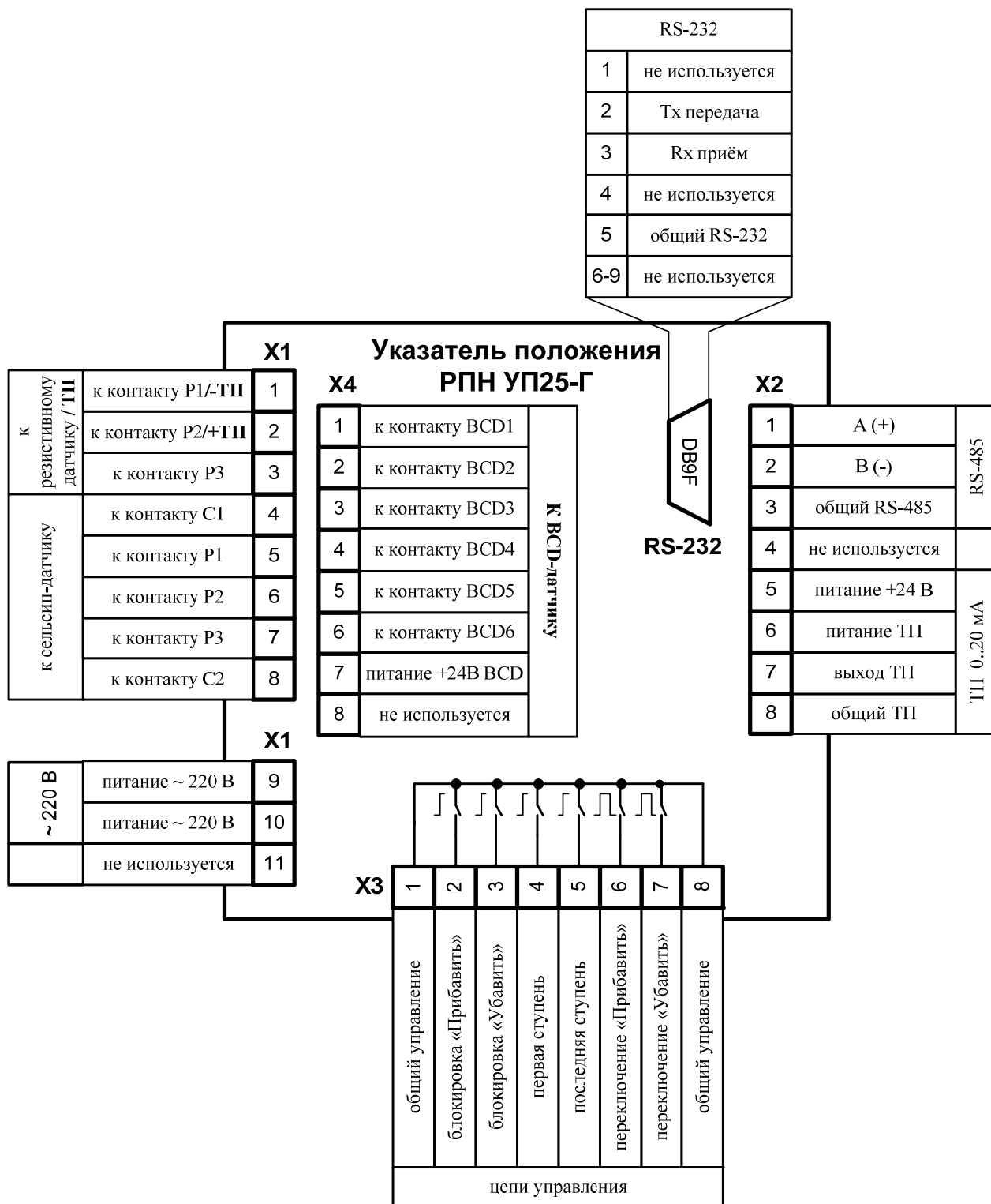
Рис. 3.1 Схема подключения УП 25-Г
