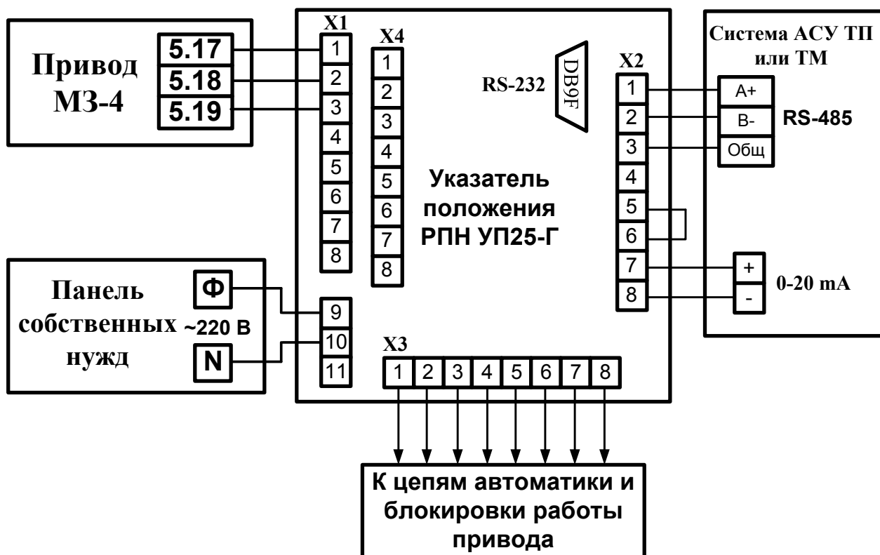
Рис. 4.2 Схема привязки УП 25-Г к приводу типа МЗ-2, МЗ-4.
