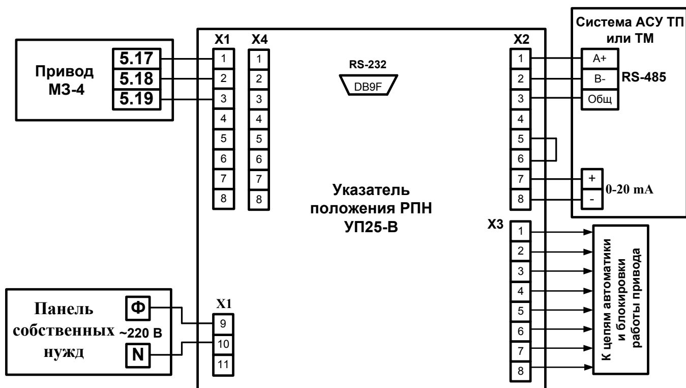
Рис. 4.2 Схема привязки УП 25-В к приводу типа МЗ-2, МЗ-4.
