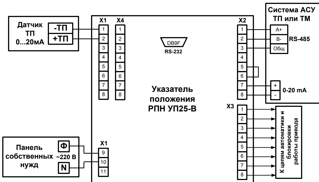
Рис. 4.3 Схема привязки УП 25-В к датчику «токовая петля» 0-20 мА.
