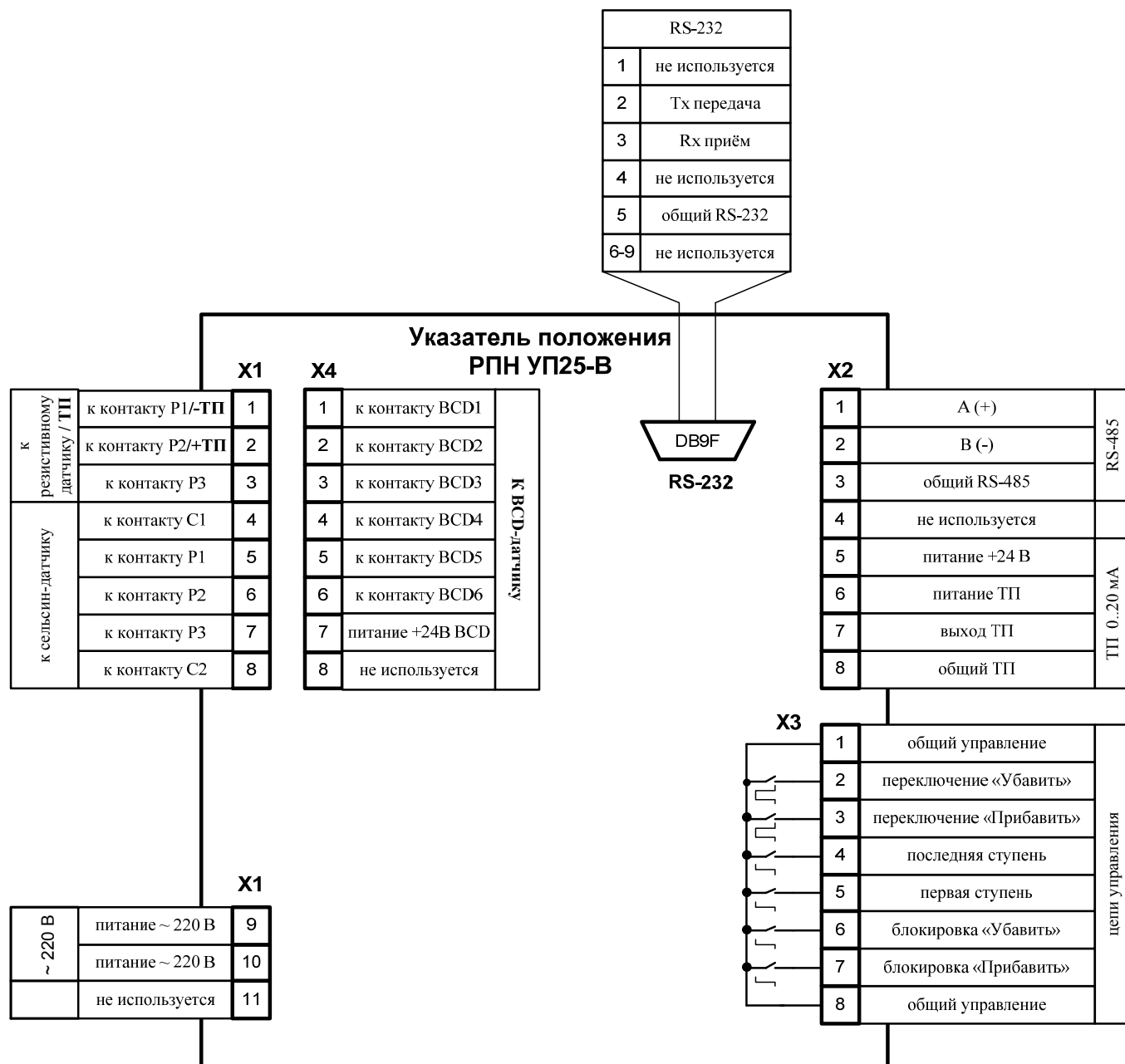
Рис. 3.1 Схема подключения УП 25-В
