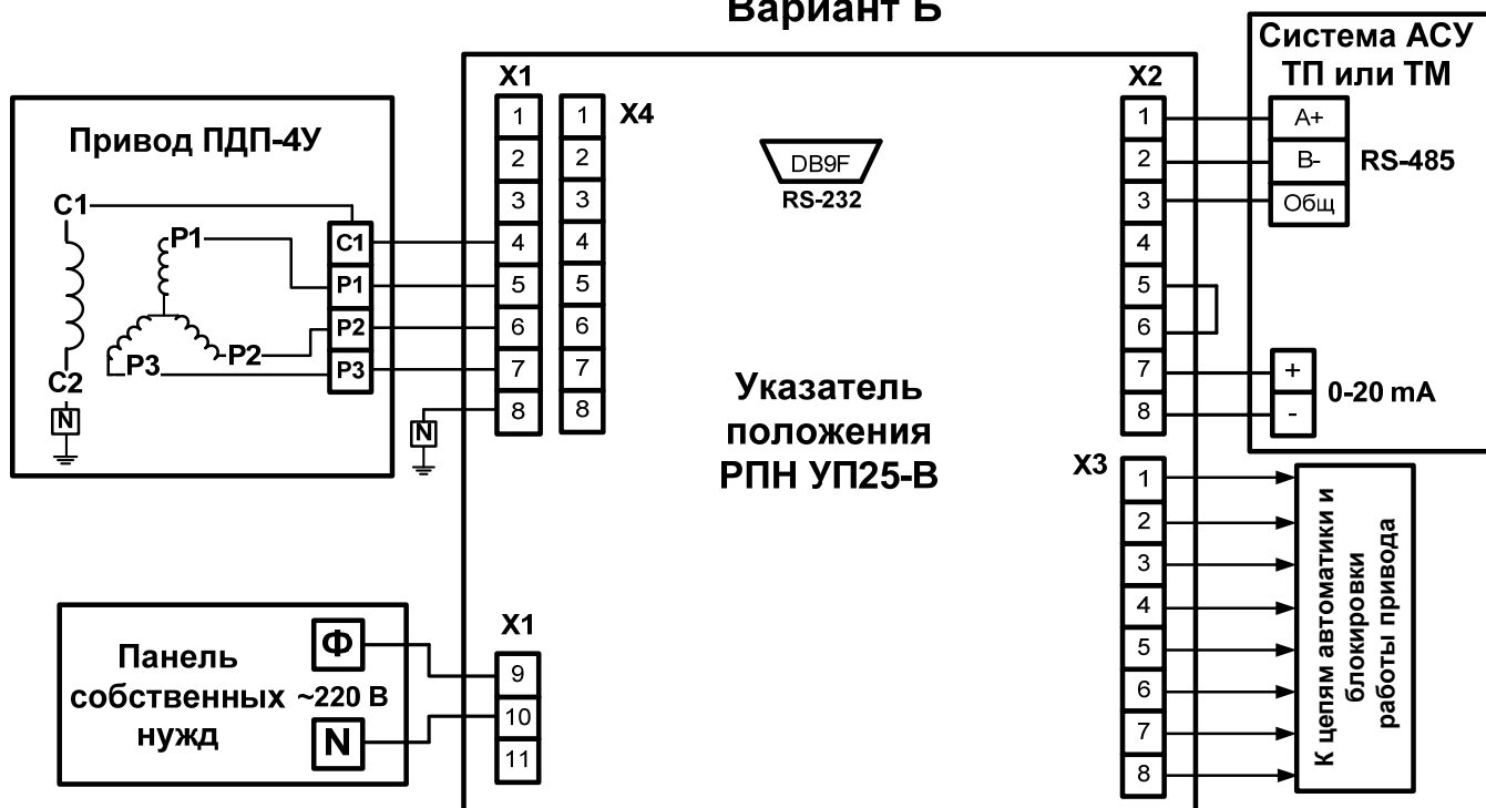
Рис. 4.1 Схемы привязки УП 25-В к приводу типа ПДП-4У.
