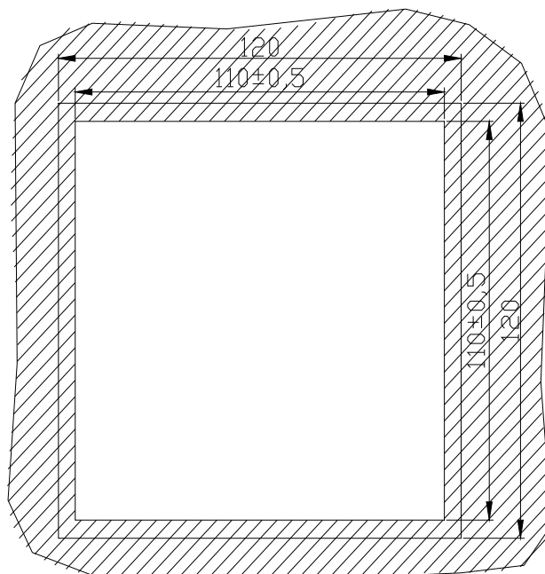
Рис. 2.2 Размеры вырубного окна в щите для установки щитового варианта указателя положения УП 25-В
