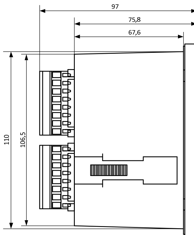
Рис. 1.1 Габаритные размеры щитового варианта указателя положения РПН УП 25-В
