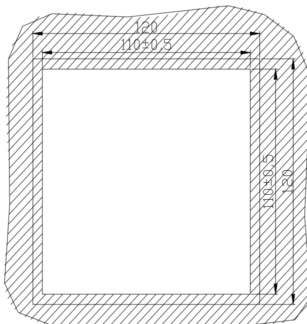
Рис. 2.2 Размеры вырубаемого окна в щите для установки щитового варианта указателя положения УП 31-Г с промежуточной рамкой
