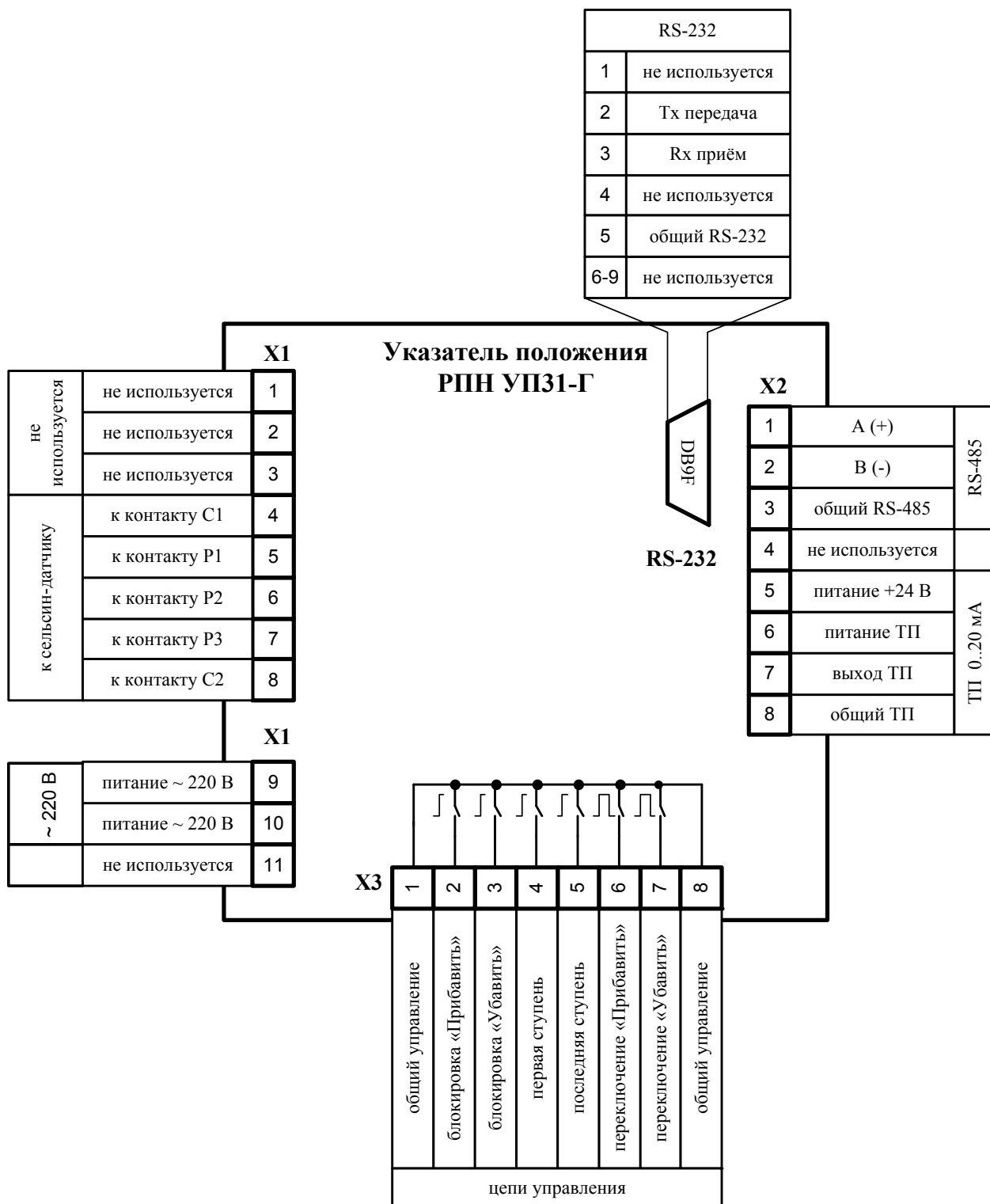
Рис. 3.1 Схема подключения УП 31-Г
