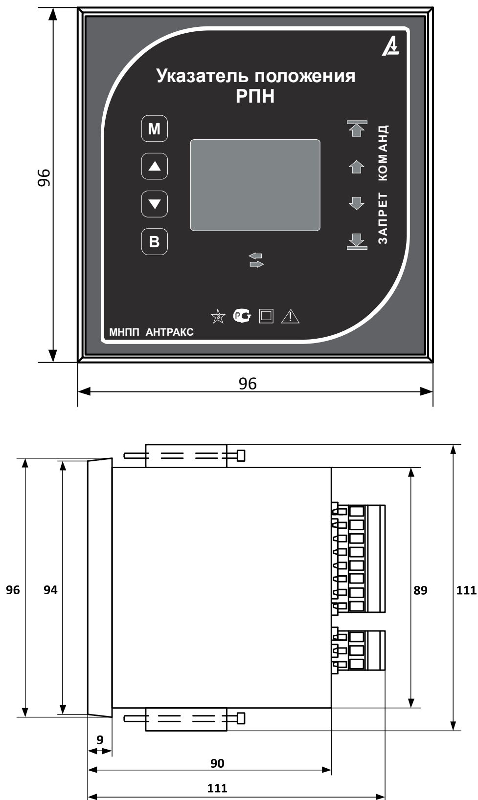
Рис. 1.1 Габаритные размеры настенного варианта указателя положения РПН УП 31-Г
