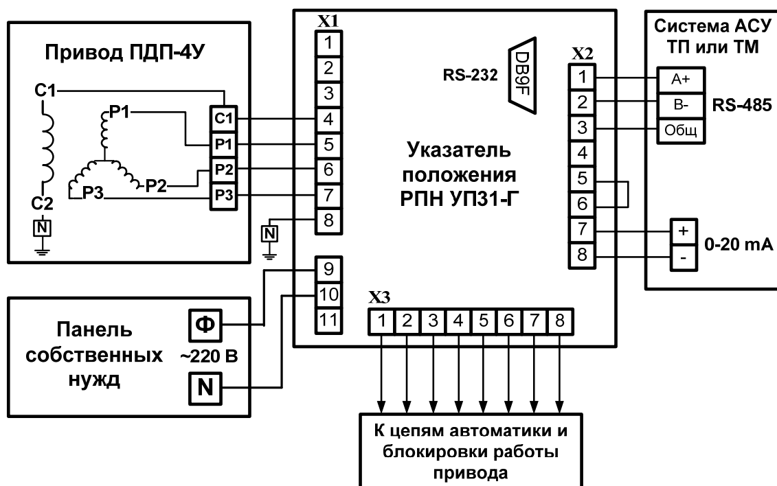
Рис. 4.1 Схемы привязки УП 31-Г к приводу типа ПДП-4У
