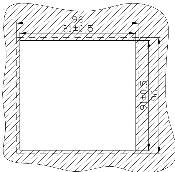
Рис. 2.1 Размеры вырубаемого окна в щите для установки щитового варианта указателя положения УП 31-Г
