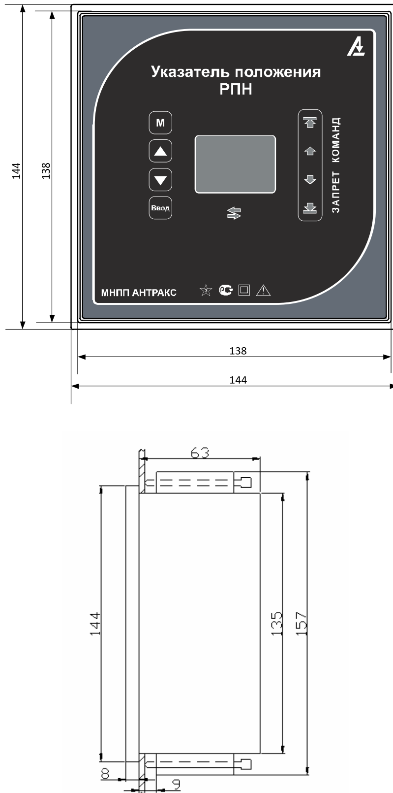
Рис. 1.1 Габаритные размеры настенного варианта указателя положения РПН УП 32-Б
