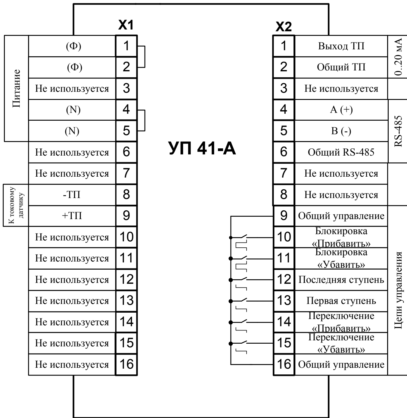
Рис. 3.1 Схема подключения УП 41-А
