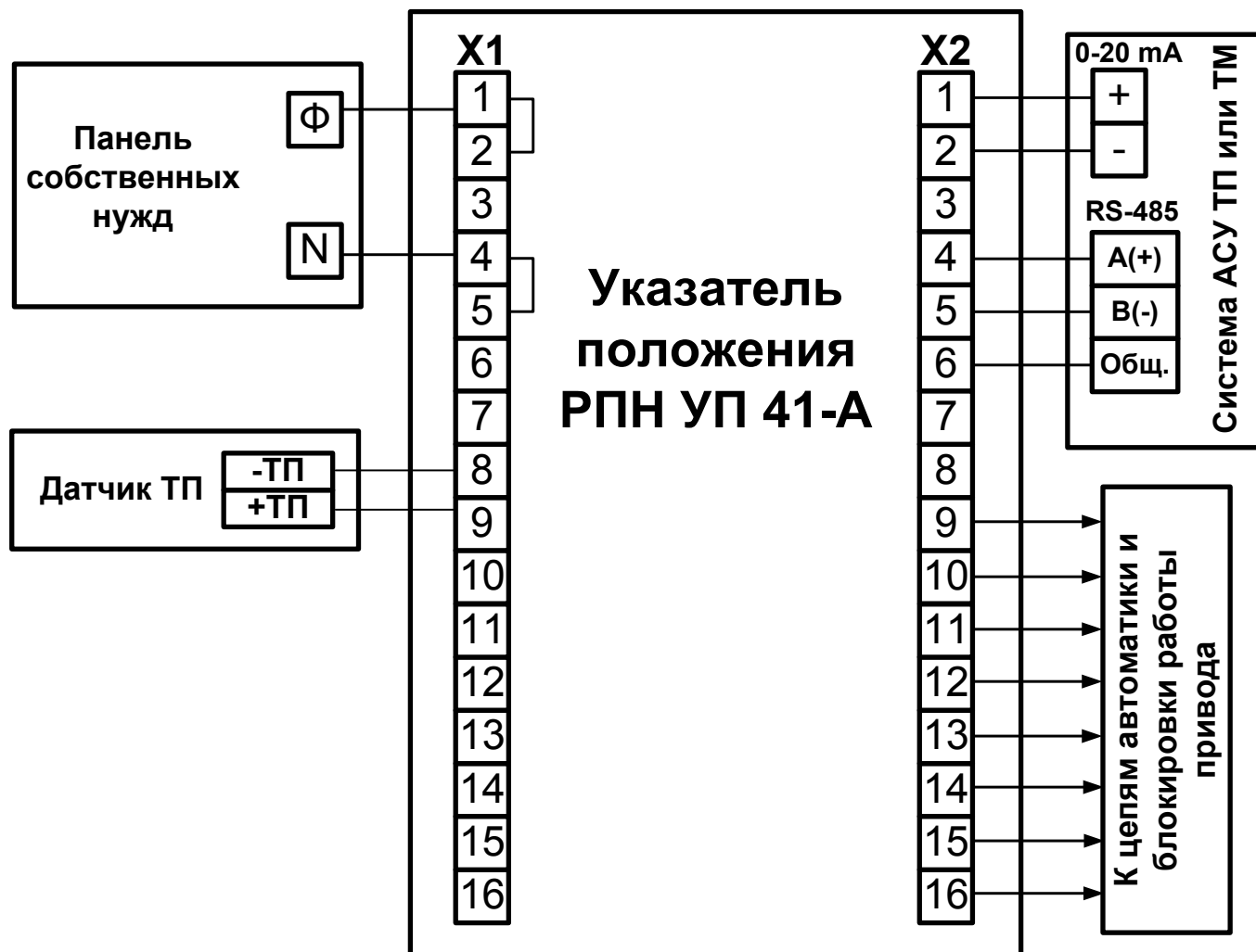
Рис. 4.1 Схема привязки УП 41-А к приводу типа MR.
