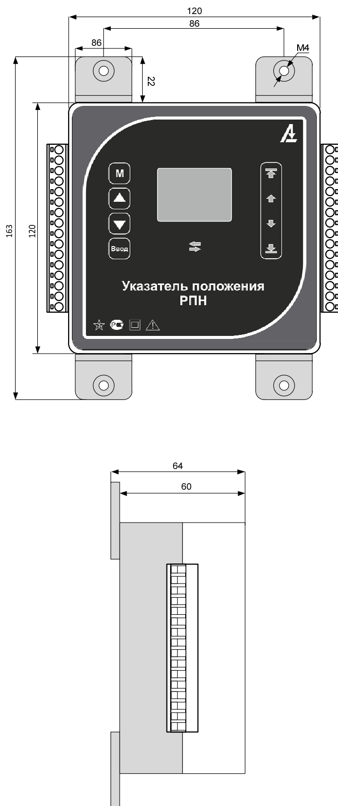
Рис. 1.1 Габаритные размеры щитового варианта указателя положения РПН УП 41-А
