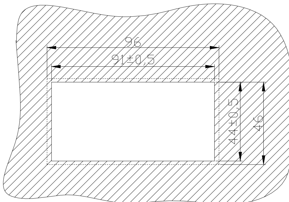
Рис. 2.1 Размеры вырубного окна в щите для установки щитового варианта указателя положения УП 41-Е
