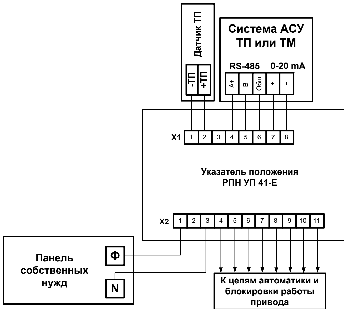
Рис. 4.1 Схема привязки УП 41-Е к приводу типа MR.
